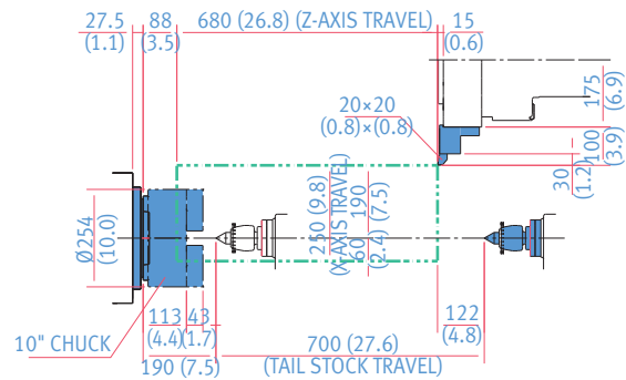
OD HOLDER
